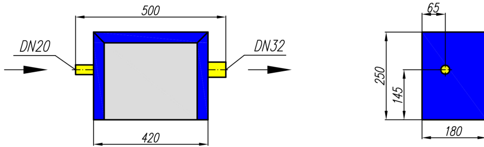
Принципиальная схема
