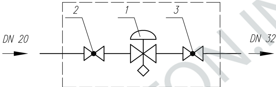
Принципиальная схема
